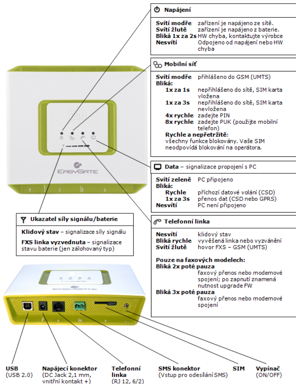
Indikační prvky EasyGate a Konektory EasyGate
