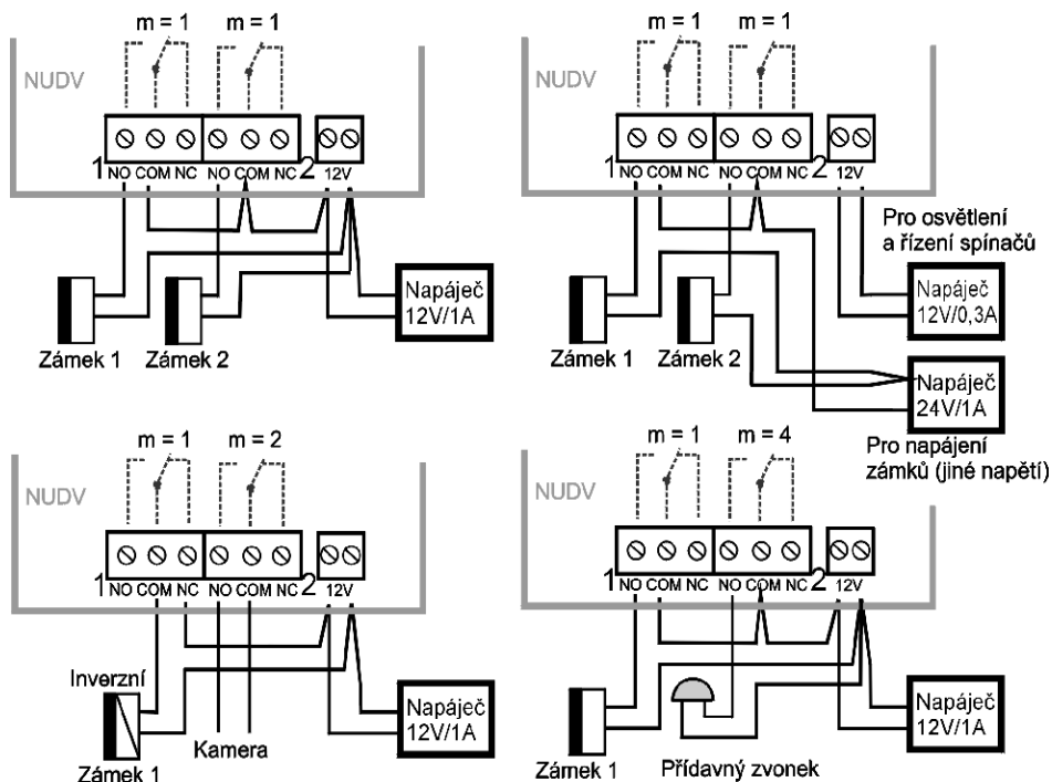
Obr. 2 Příklady zapojení spínačů
