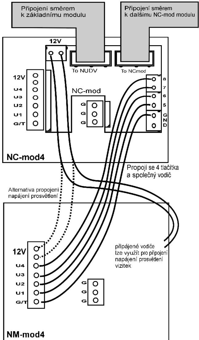
Obr. 3 Propojení NC-mod a NM-mod
