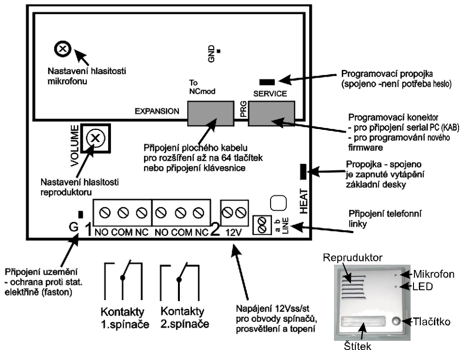
Obr. 1 Pohled zezadu na základní modul
